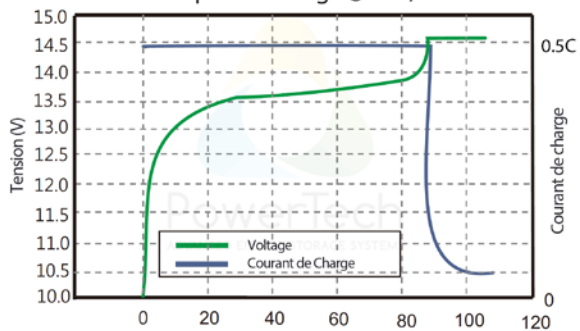
Caractéristiques de charge @0.5C, 25°C
